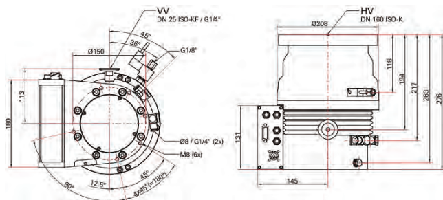
HiPace 700M
