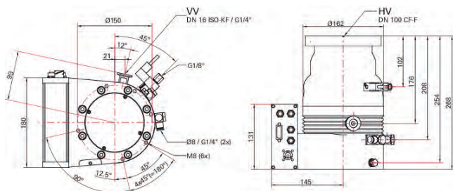
HiPace 300M
