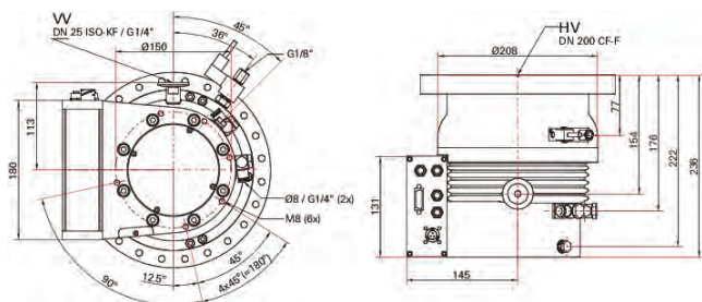
HiPace 800M
